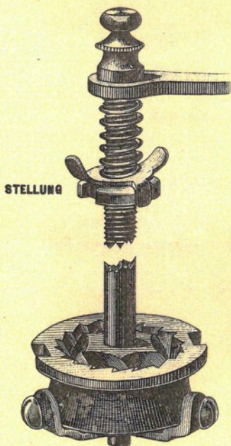
Mahlwerk der „Ideal“-Kaffeemühle mit äusserer Stellung.
