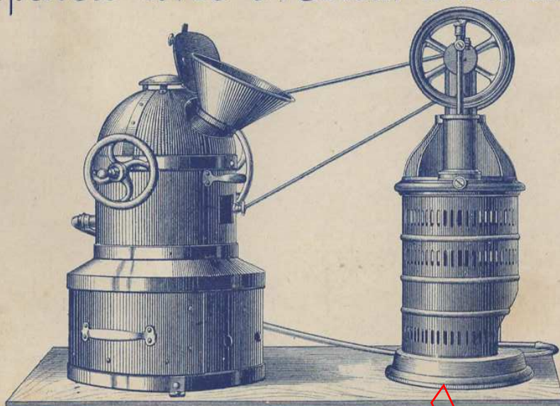
Modèle d'une Installation de Brûloir à Gaz, avec Moteur à air chaud de 1/30 e Radiateur, le tout monté sur tablette en chêne de 120 x 35
