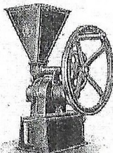
Tischmühle Modell S für Handbetrieb. Teleg.-Wort: Soris RM.
