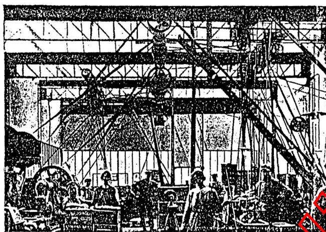
Atelier de Mécanique Fraisage et taillage des broyeurs
